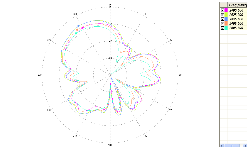
E2-Plan [Vertical]
