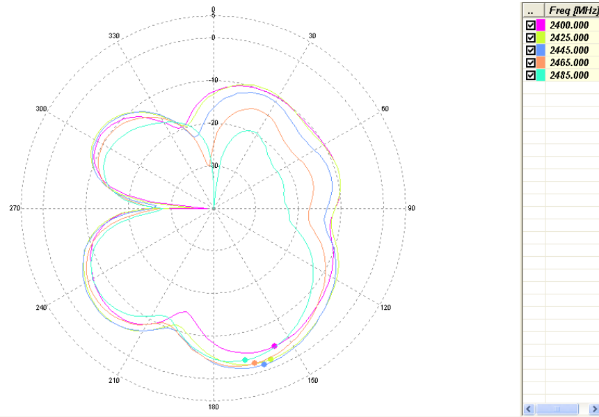
H-Plan [Vertical]
