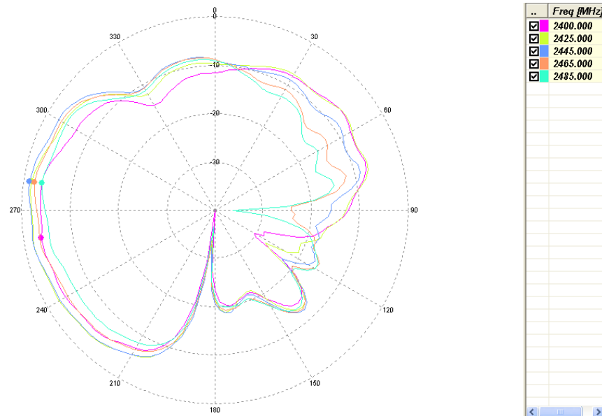
E1-Plan [Vertical]
