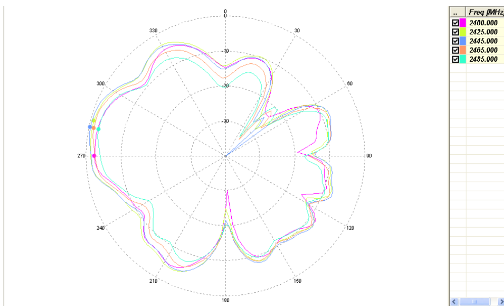
E1-Plan [Horizontal]
