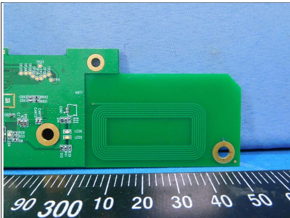
NFC Antenna
