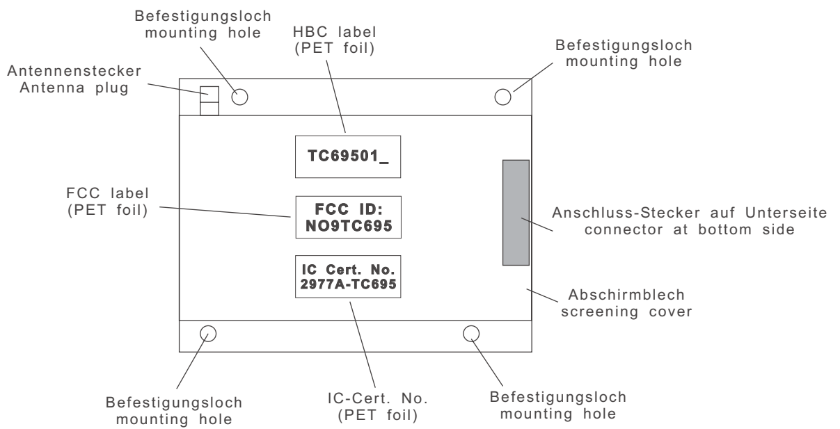
Skizze M1:1 scale 1:1
