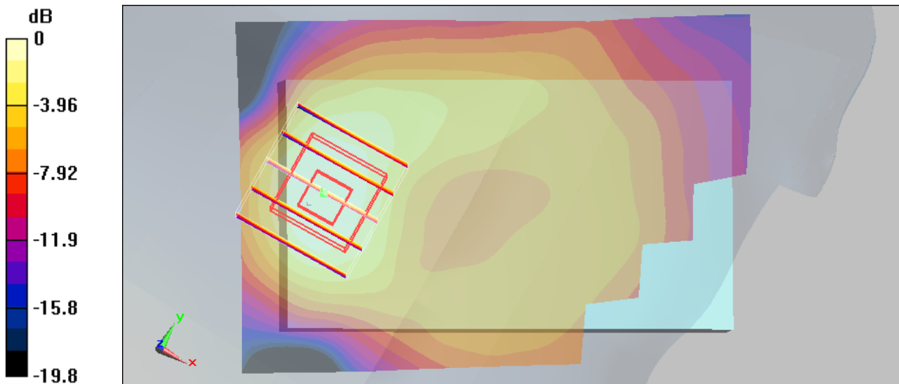
0 dB = 0.108mW/g
