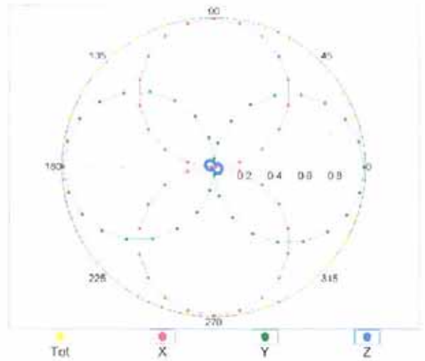
f=2500 MHz,R22,0°
