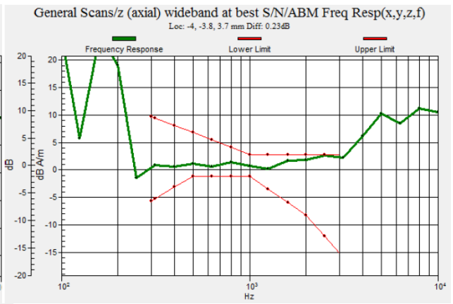
Fig 9.4 CDMA2000 BC1 Ch25
