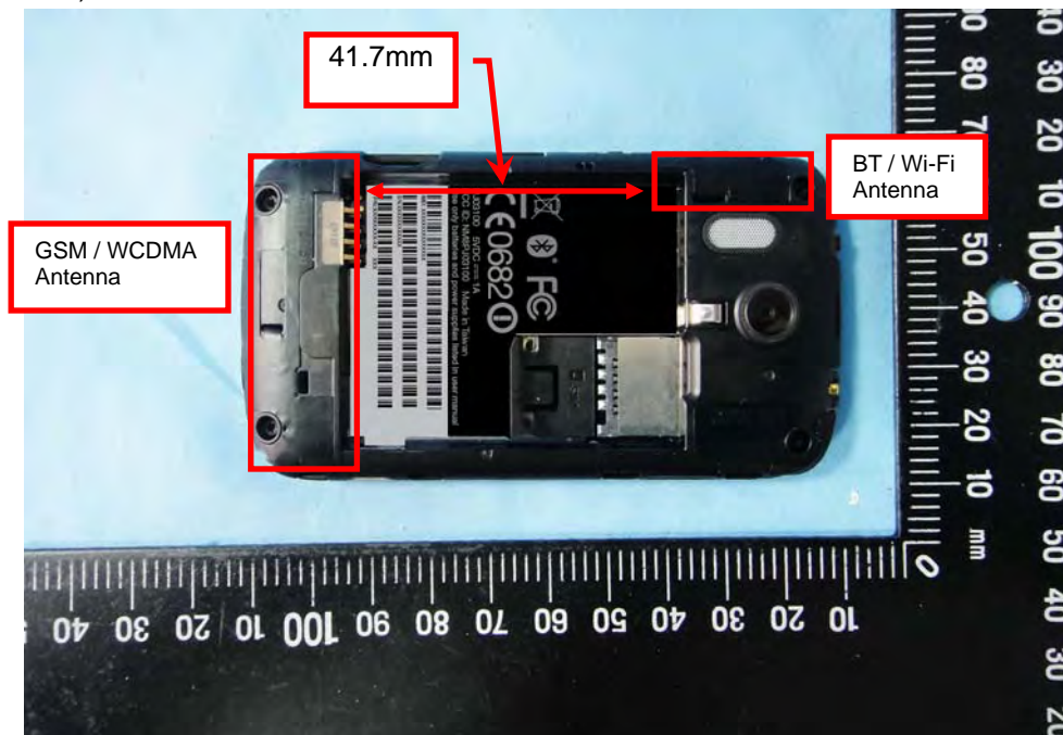
EUT Photo 2 )
