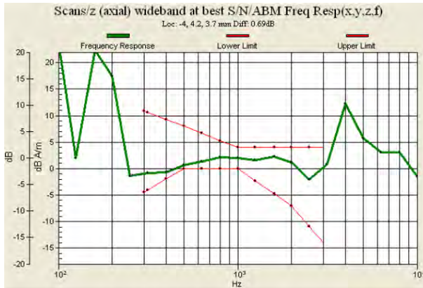
Fig. 9.7 GSM1900 Ch810
