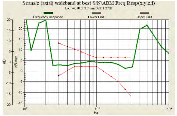
Fig. 9.4 GSM850 Ch251
