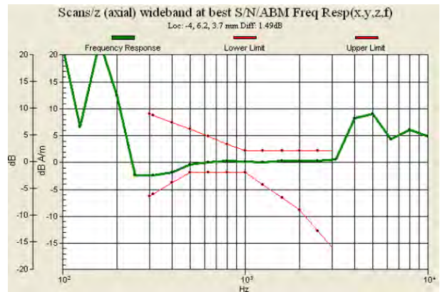
Fig. 9.10 WCDMA Band V Ch4182
