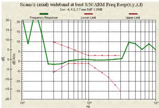
Fig. 9.9 WCDMA Band V Ch4132
