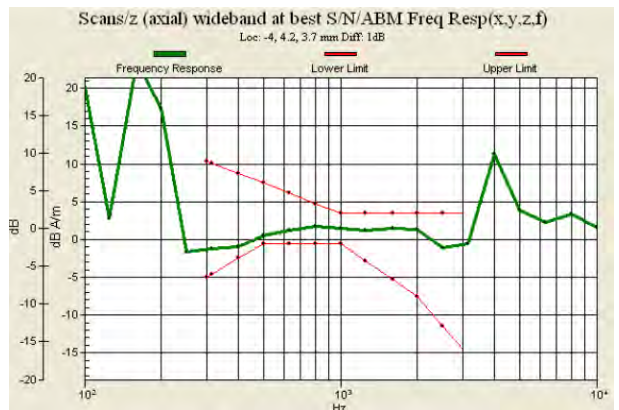
Fig. 9.6 GSM1900 Ch661
