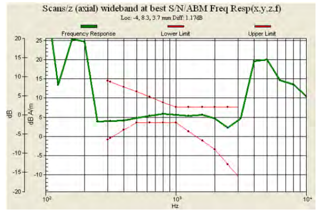
Fig. 9.8 GSM1900 Ch810
