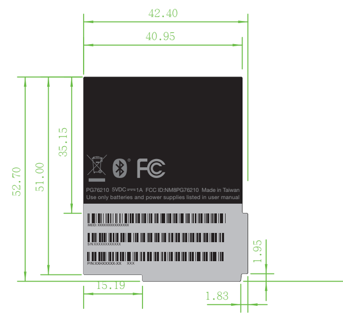
前視圖2
