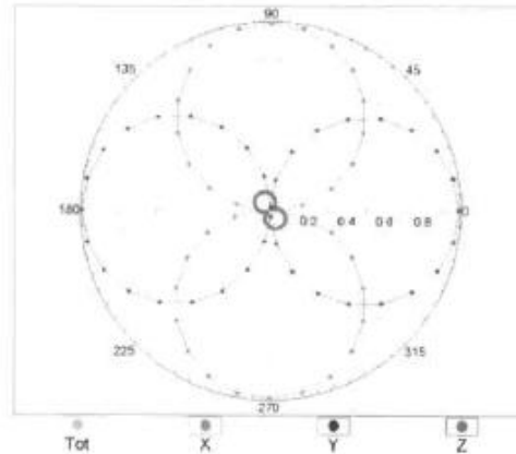
f=2500 MHz,R22,0°
