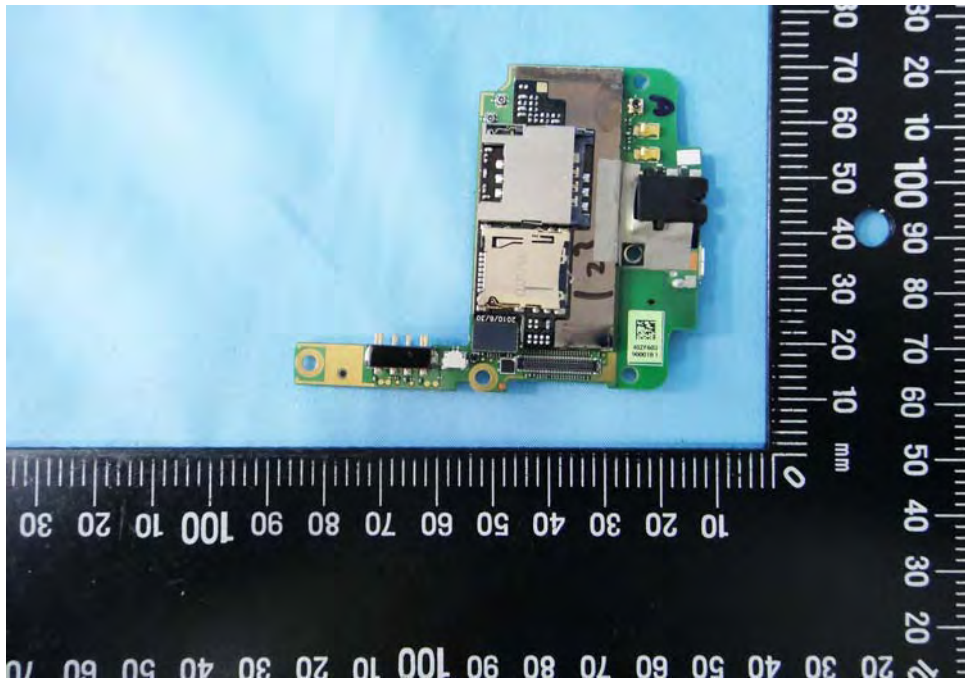
EUT Photo 10 )
