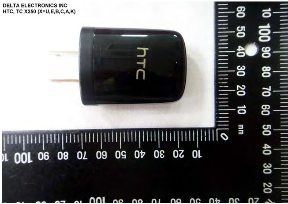
EUT Photo 12 )
