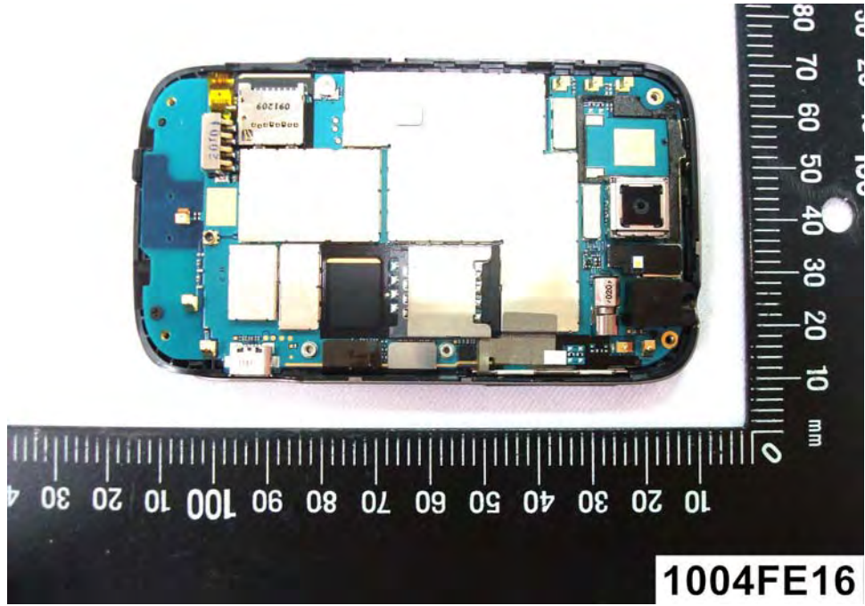
(9) EUT Photo
