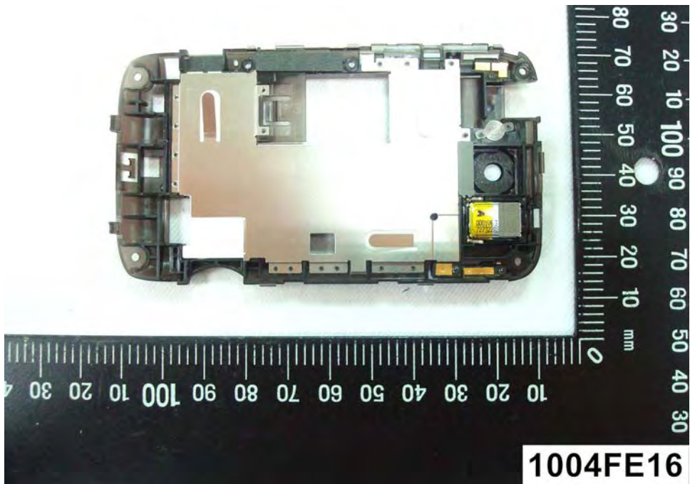
(8) EUT Photo
