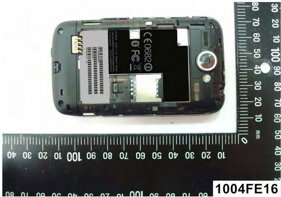
(2) EUT Photo
