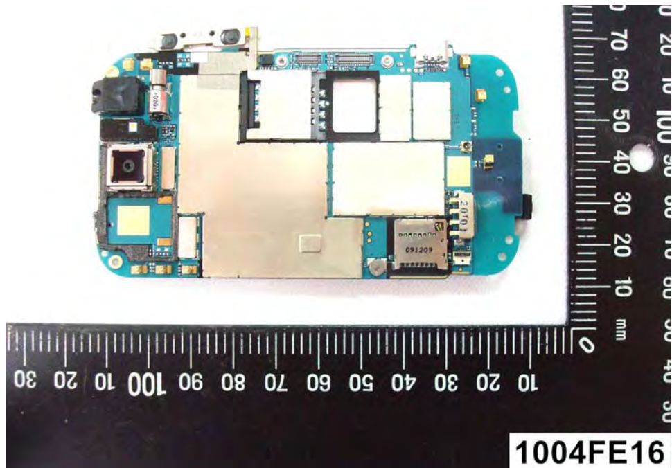
(10) EUT Photo
