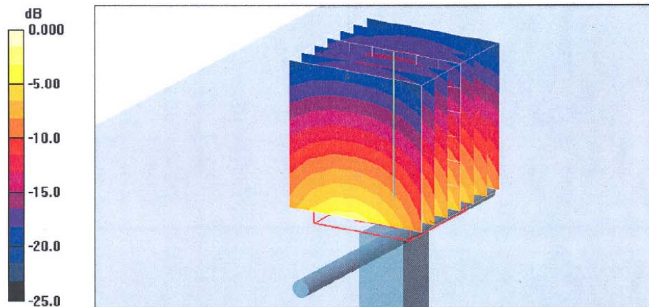
0 dB = 15.0mW/g
