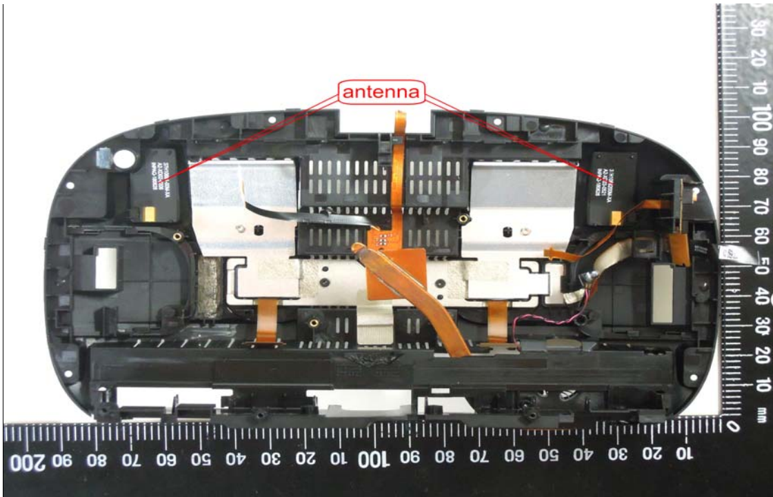
Antenna
