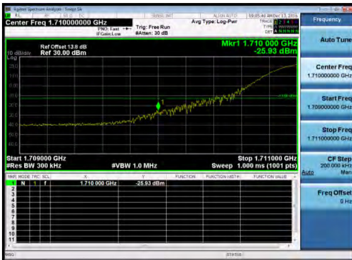
Band Edge_Band4_20MHz_QPSK_1_0_LowCH20050-1720
