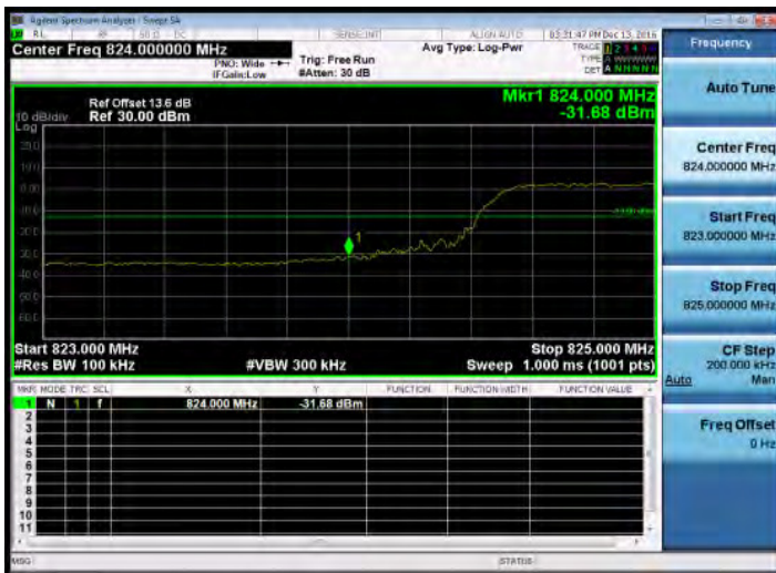
Band Edge_Band5_10MHz_QPSK_50_0_LowCH20450-829
