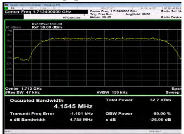
WCDMA_B4_LowCH1312-1712.4
