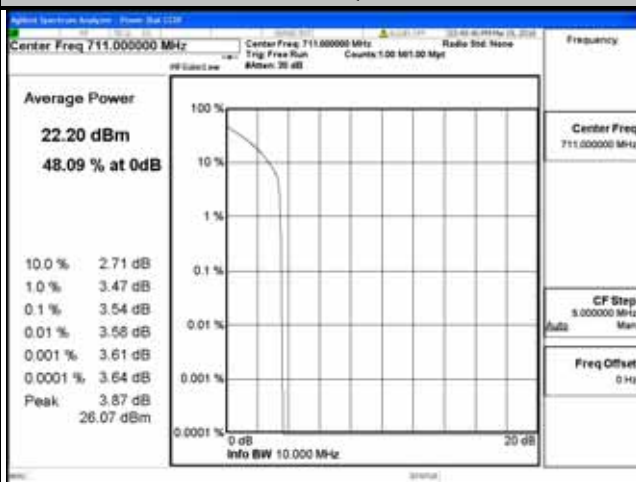
10 MHz / QPSK
