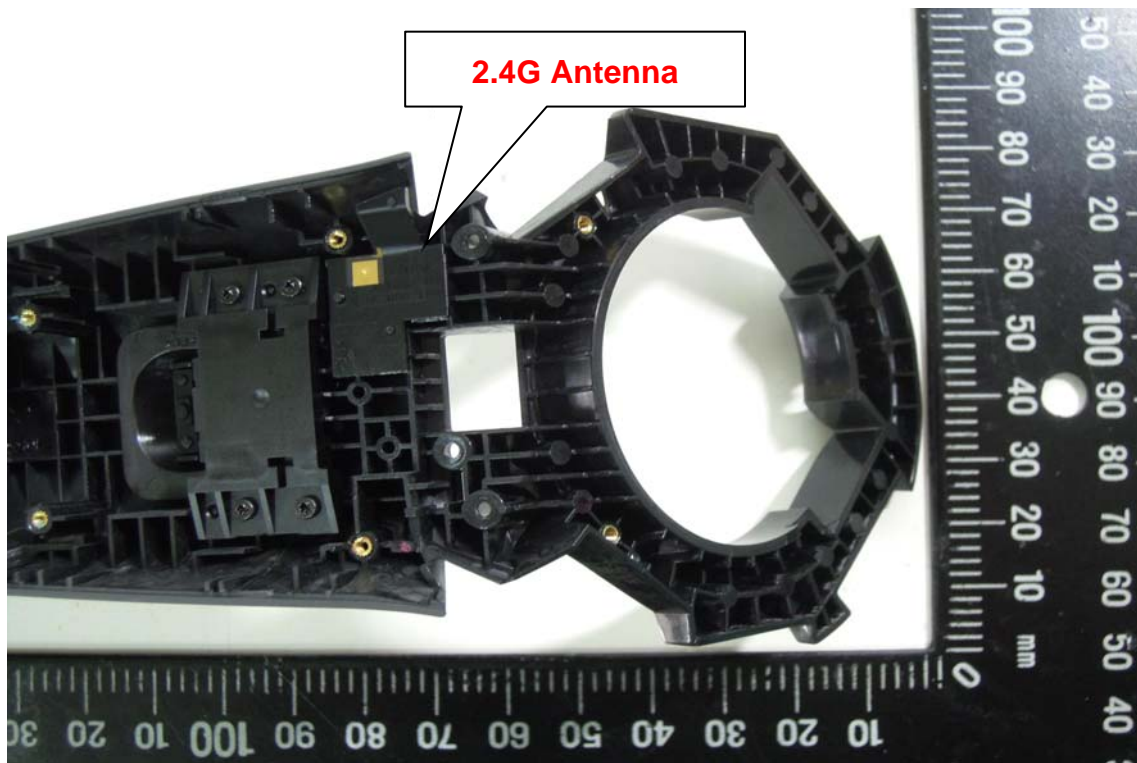
2.4G Antenna
