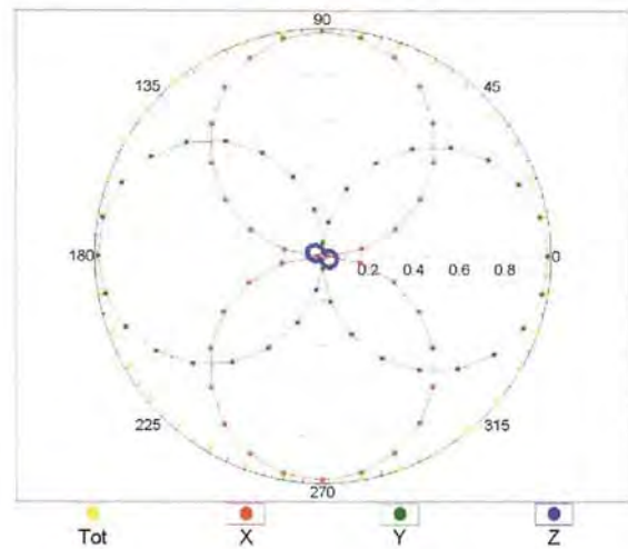
f=2500 MHz,R22,0°
