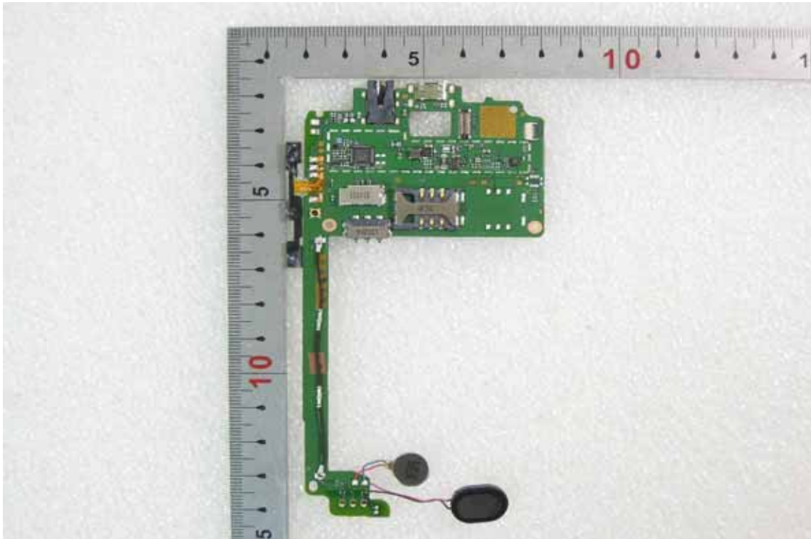
WWAN Antenna
