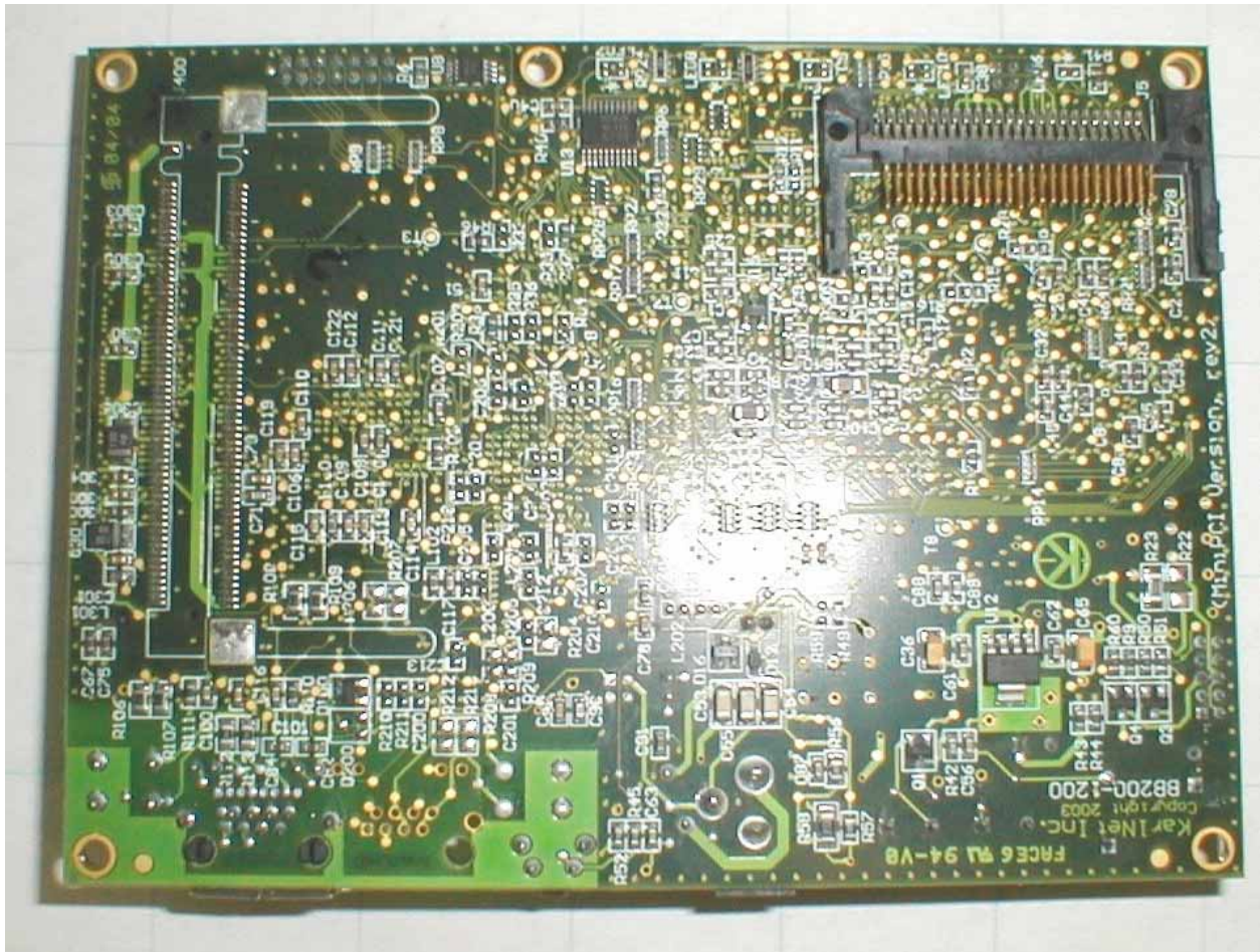
PCB Bottom
