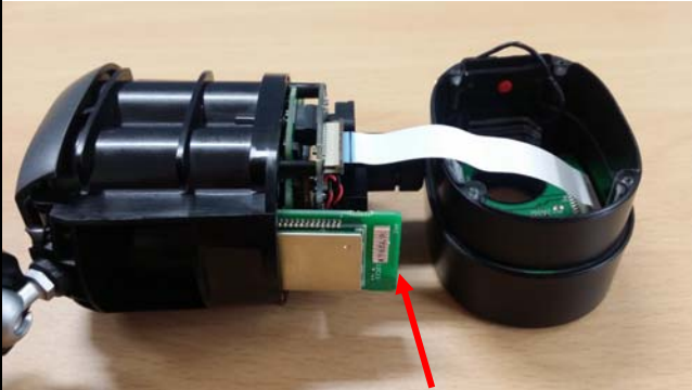
900MHz Antenna
