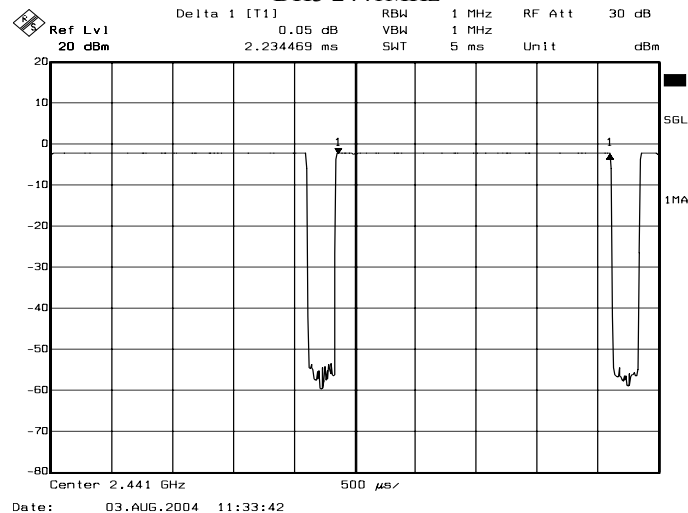
DH5 2441MHz
