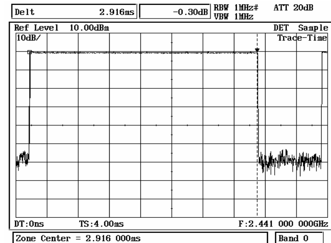
DH5 2441MHz
