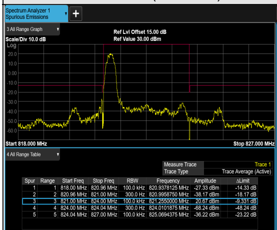
1RB#0 (822.5MHz)
