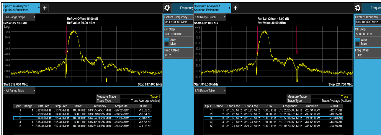
1RB#0 (814.7MHz)
