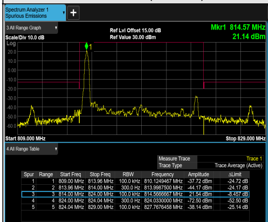
1RB#0 (819MHz)
