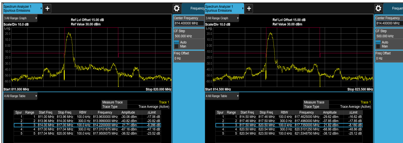
1RB#0 (815.5MHz)
