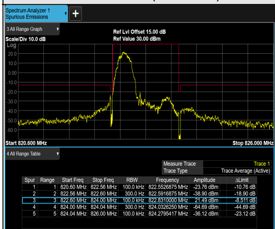
1RB#0 (823.3MHz)
