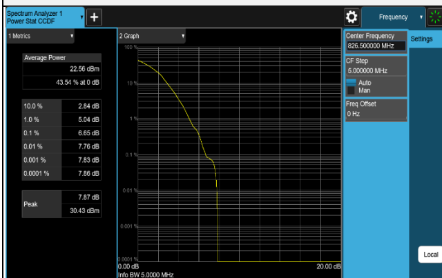
16QAM CH 20425 (826.5MHz)
