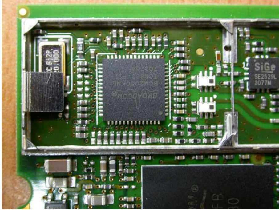
RF Module 3
