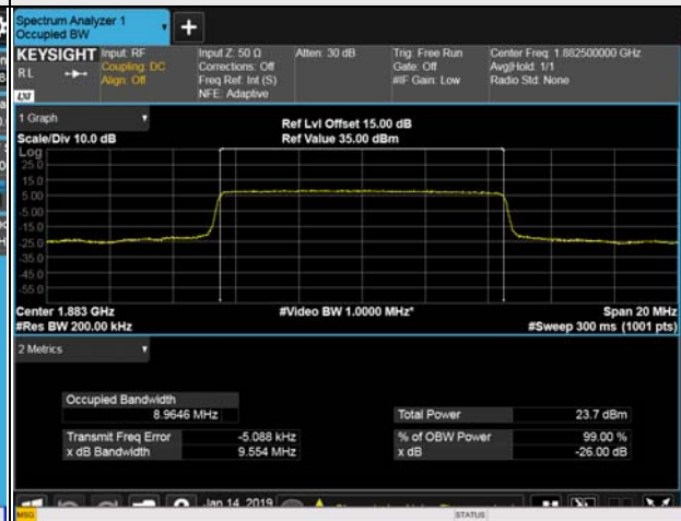
20MHz / 16QAM
