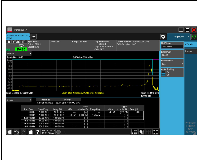
5G NR n66_CH352000_40M_pi/2 BPSK_1RB215
