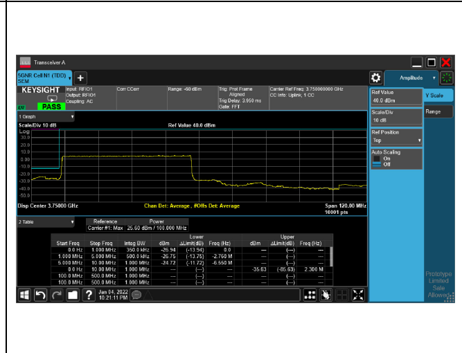
5G NR n77_CH 66366650M_pi/2 BPSK_128RB5
