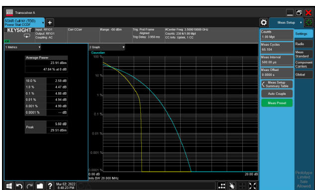
5G NR n77_CH633334_15M_1RB_QPSK_Ratio
