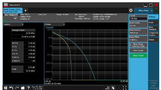
5G NR n77_CH633334_20M_1RB_16-QAM_Ratio
