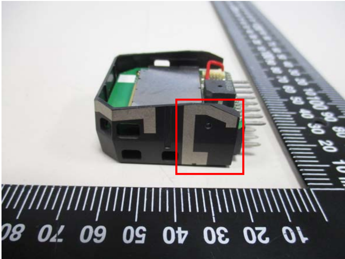
GPS antenna
