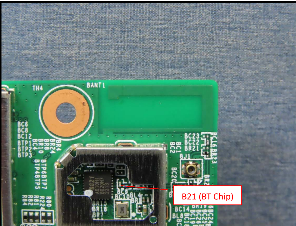
BLE ANT
