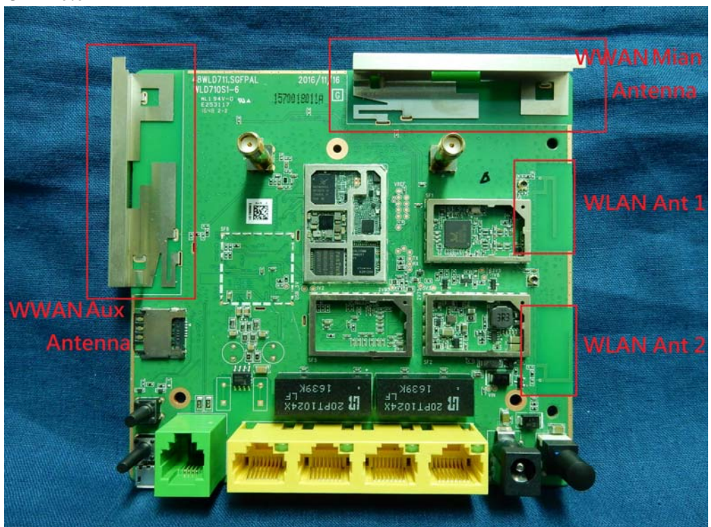
(9) EUT Photo
