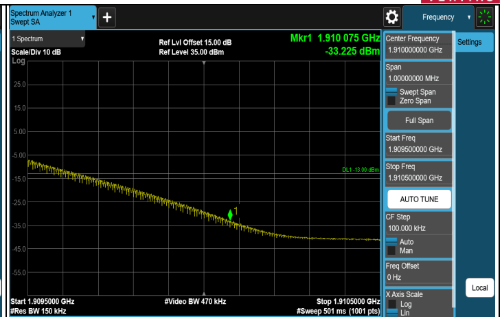
1RB (1902.5 MHz)
