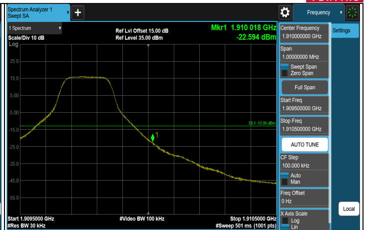
1RB (1908.5 MHz)
