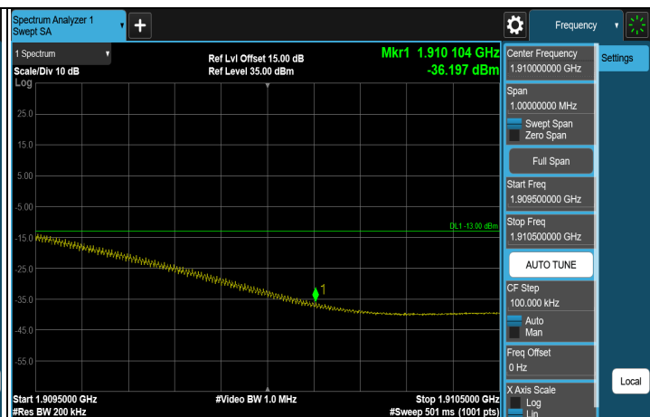
1RB (1900 MHz)
