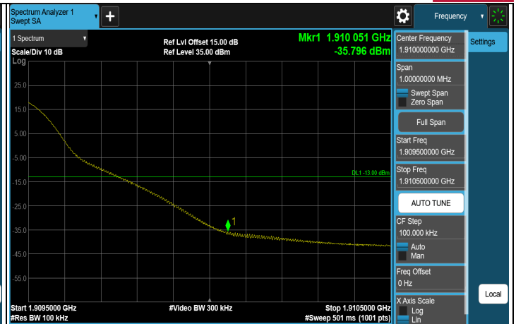
1RB (1905 MHz)
