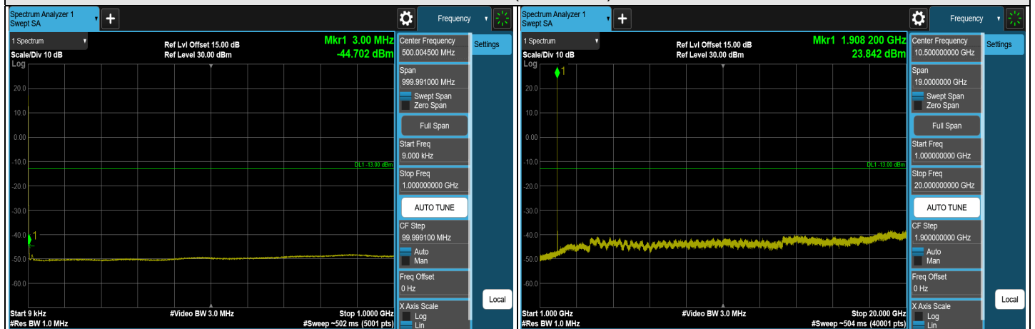
CH 19193 (1909.3 MHz)
