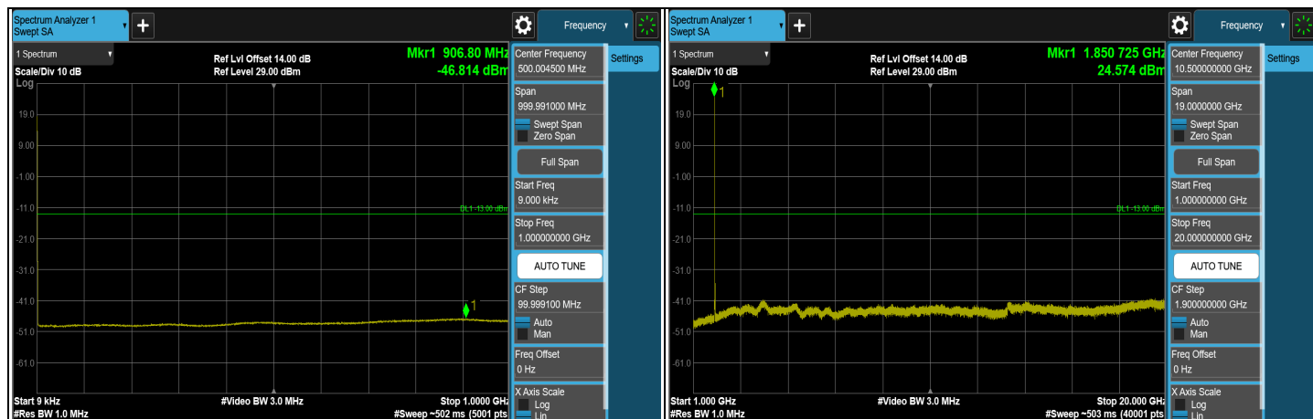
CH 2609 (1855 MHz)
