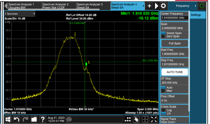
CH 810 (1909.8 MHz)
