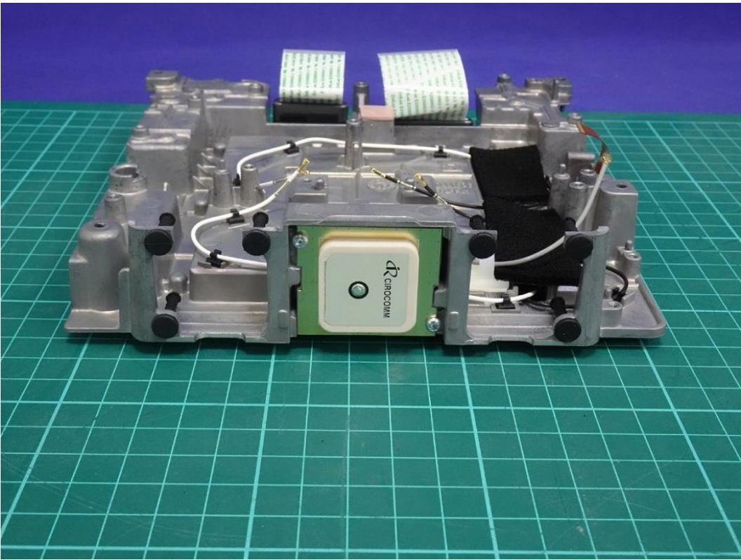
(77) EUT Photo
