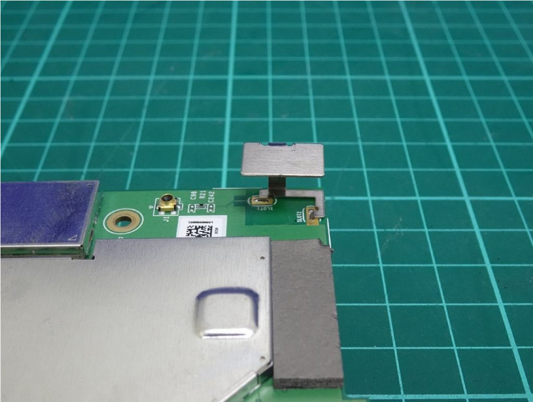
(56) EUT Photo
