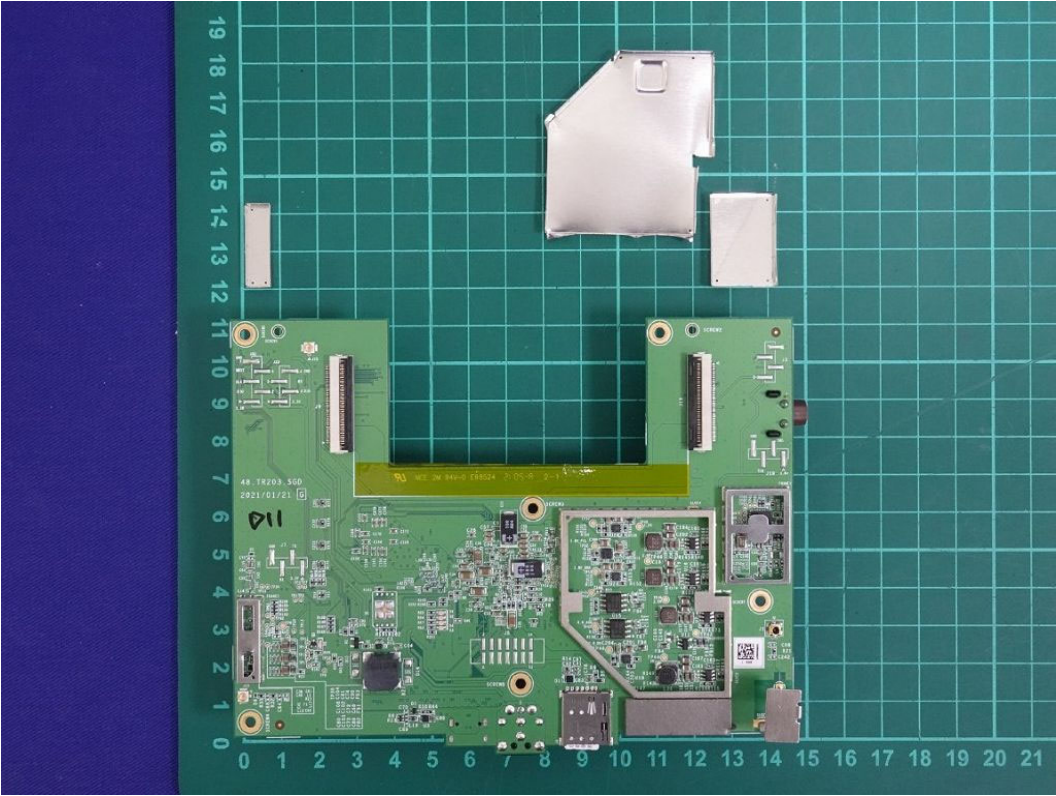
(57) EUT Photo
