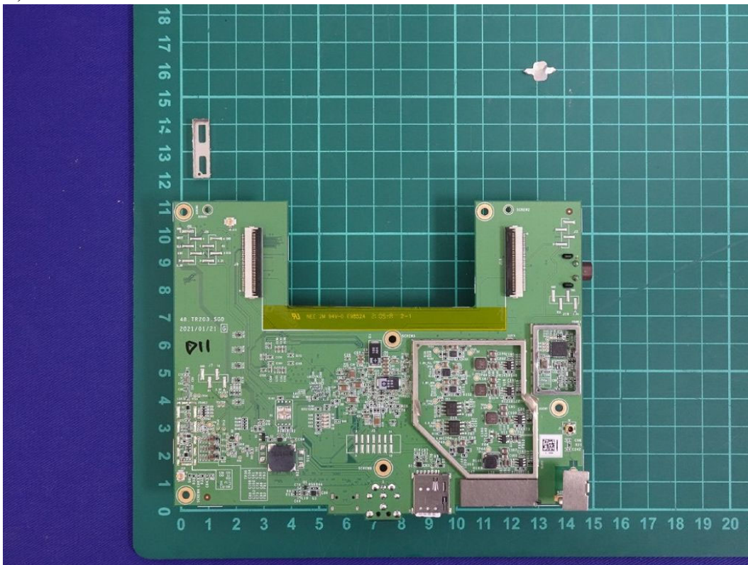
(59) EUT Photo
