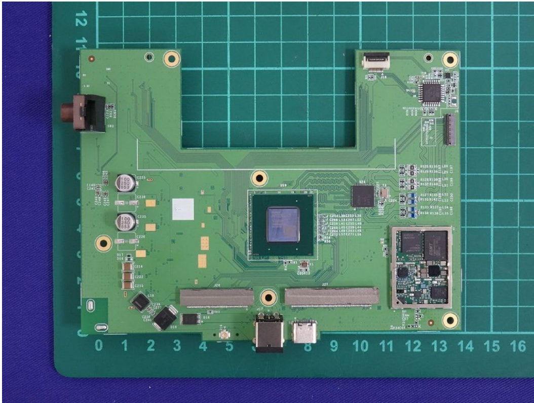
(70) EUT Photo
