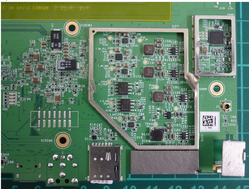
(63) EUT Photo
