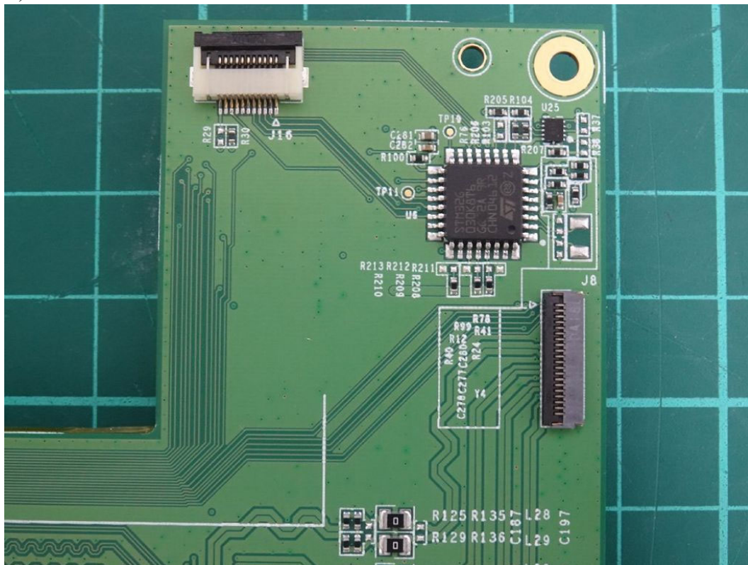
(75) EUT Photo
