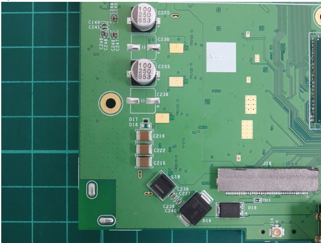
(72) EUT Photo
