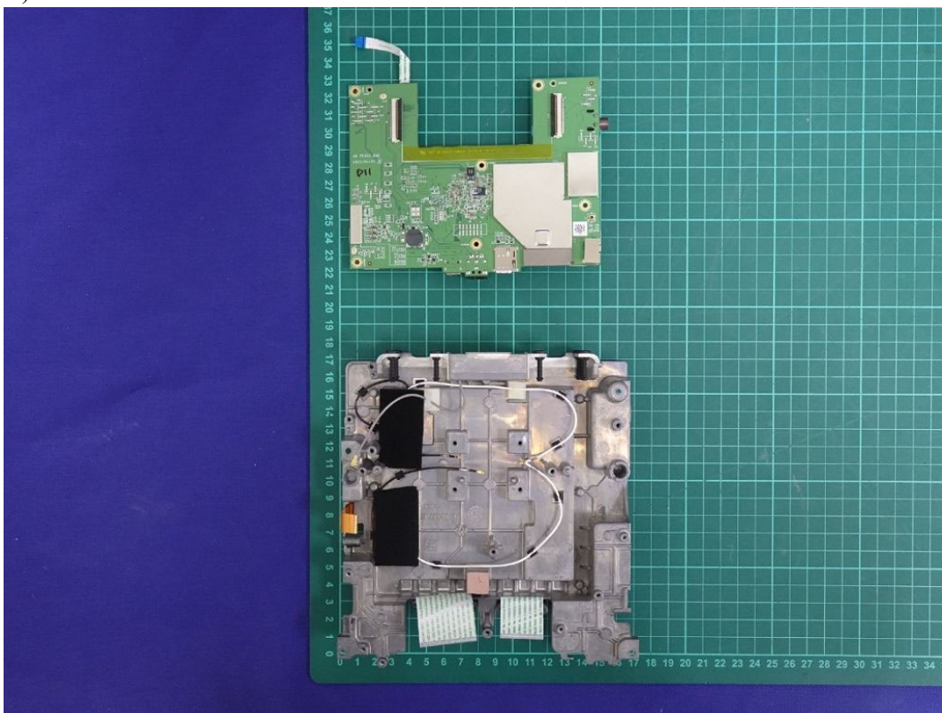
(53) EUT Photo
