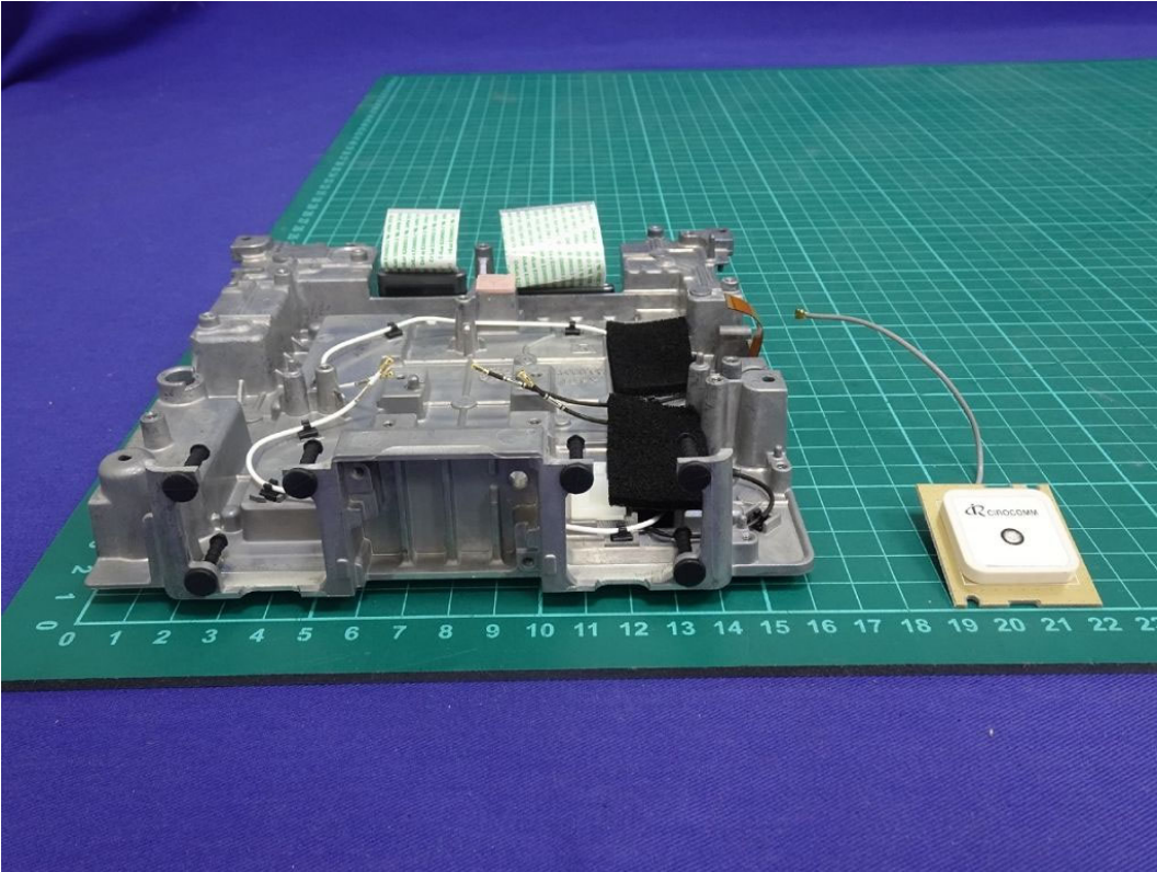
(78) EUT Photo
