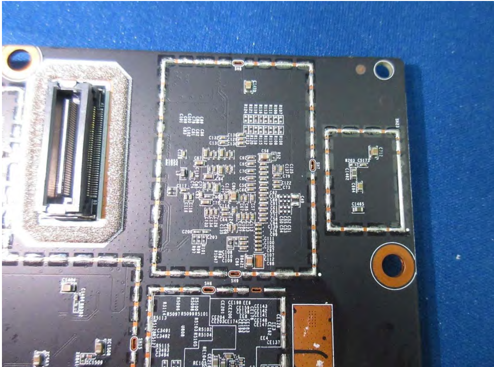
(82) EUT Photo
