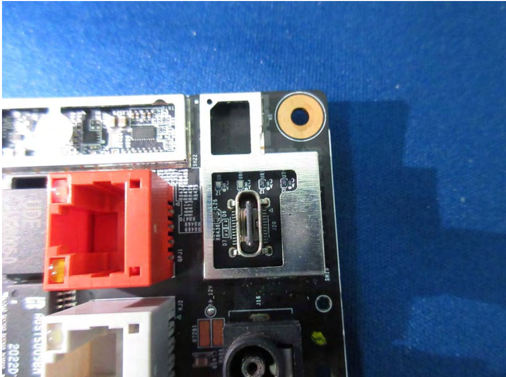
(74) EUT Photo
