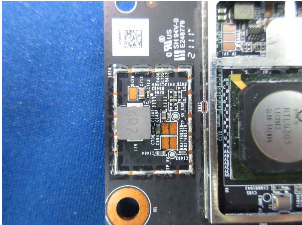
(54) EUT Photo
