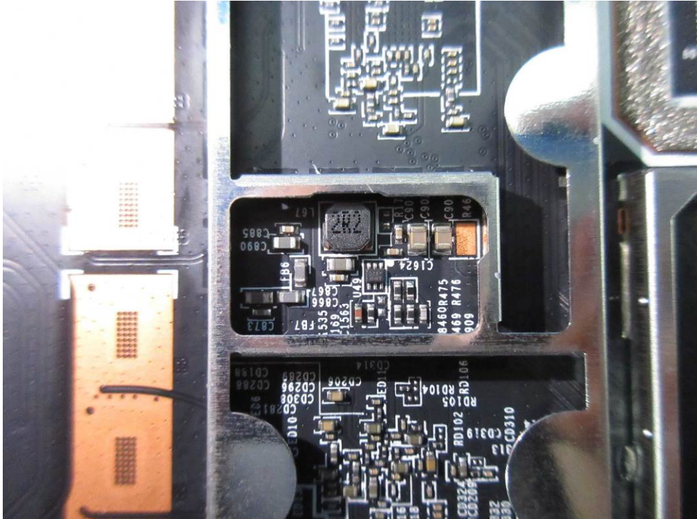
(61) EUT Photo
