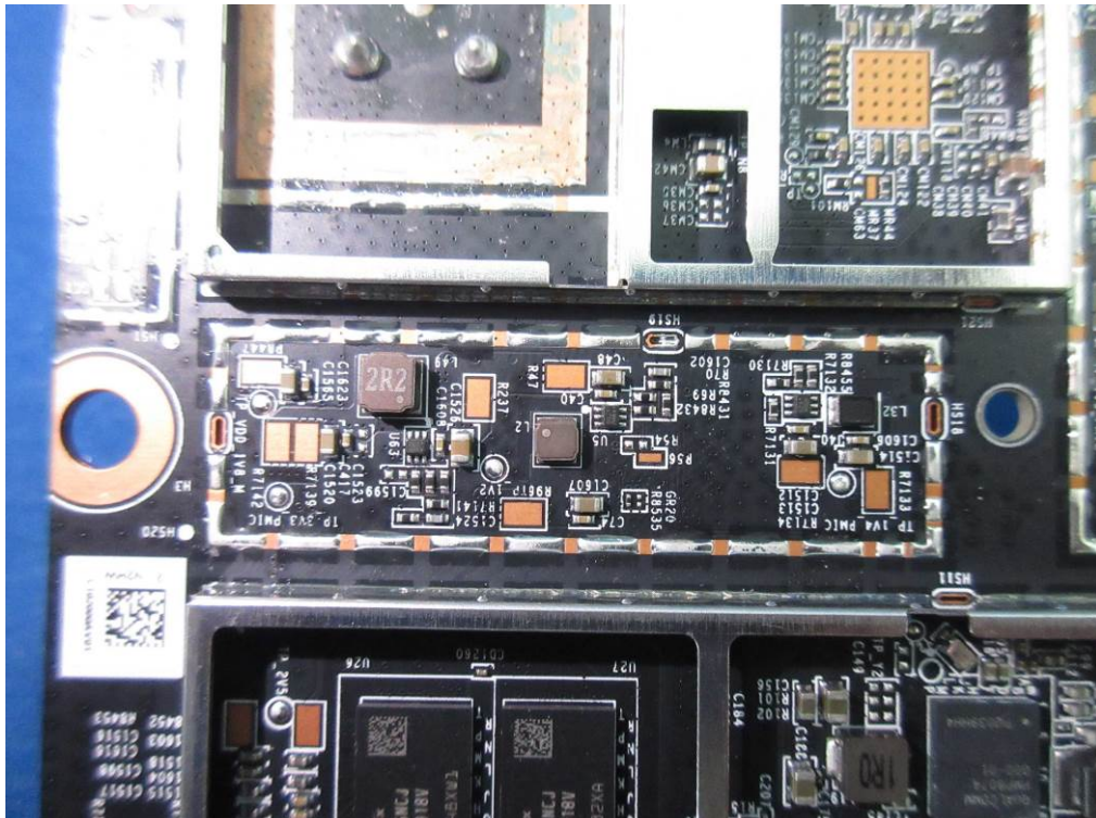
(77) EUT Photo
