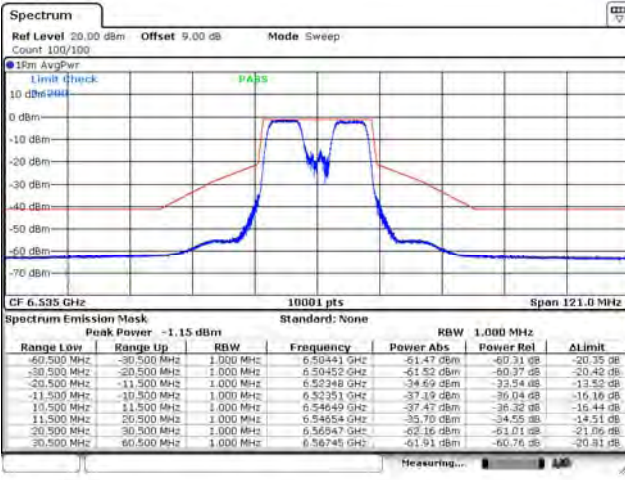
802.11ax (20 MHz) / Ant. 2 / 6535 MHz
