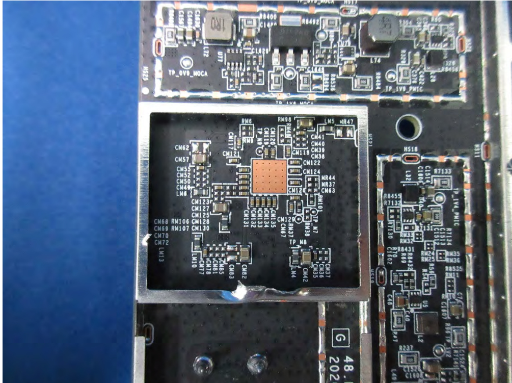
(116) EUT Photo
