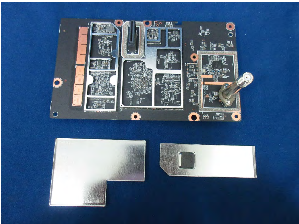
(67) EUT Photo
