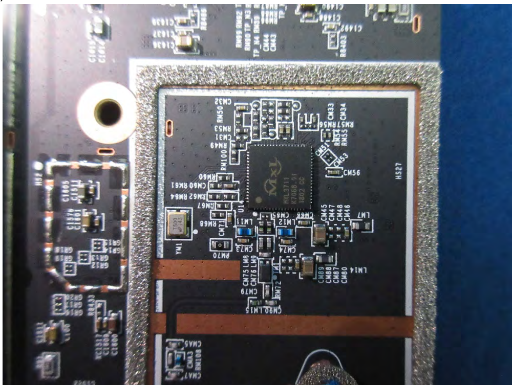
(81) EUT Photo
