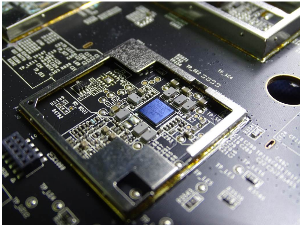
(82) EUT Photo
