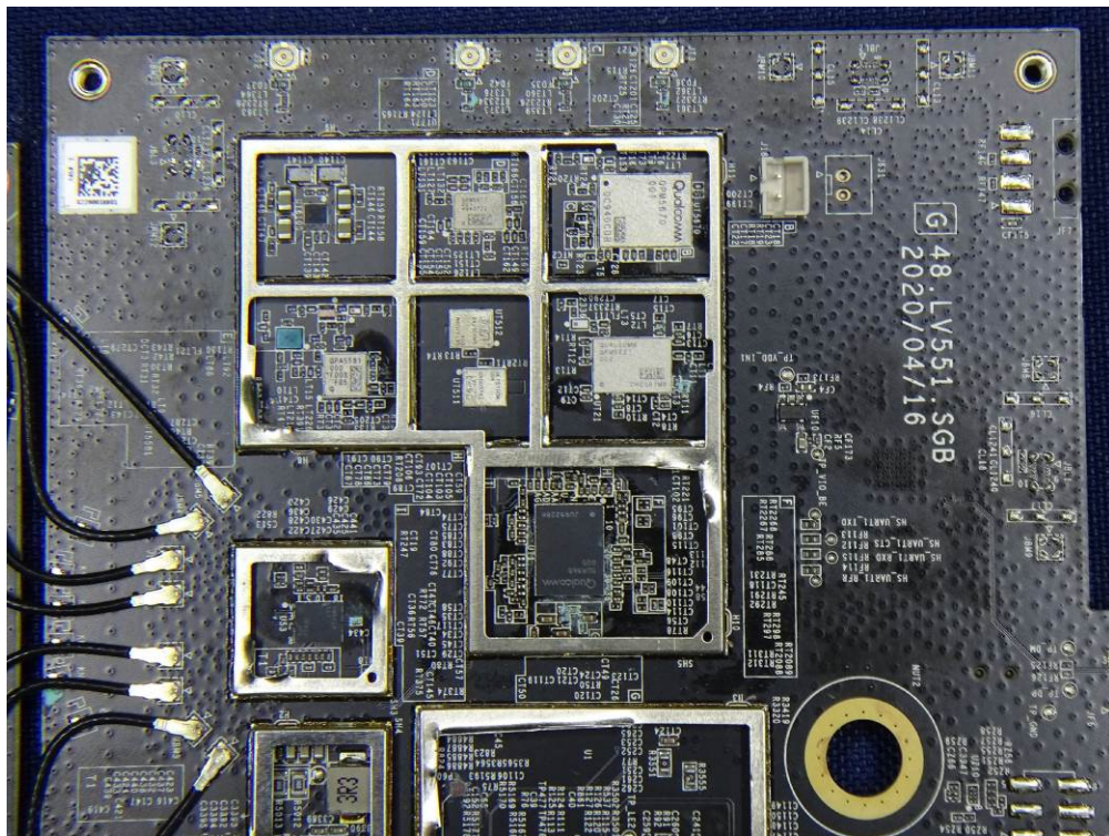
(95) EUT Photo
