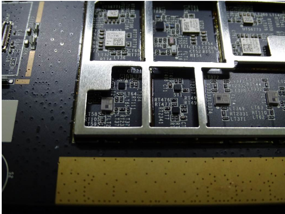
(85) EUT Photo
