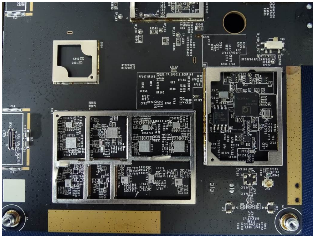
(81) EUT Photo
