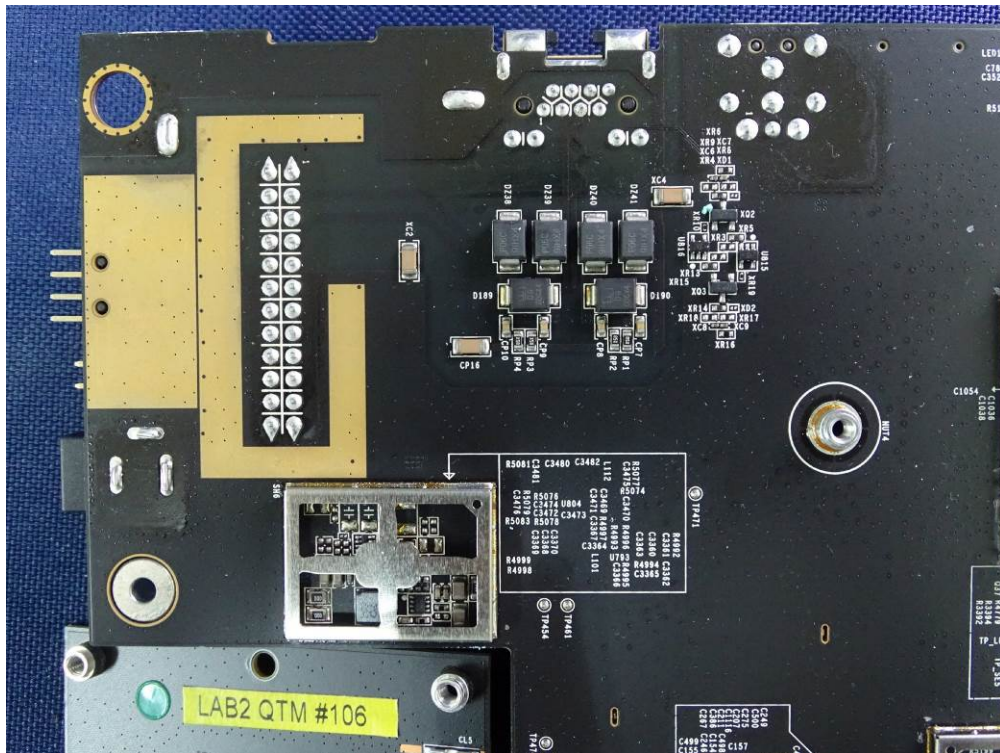
(74) EUT Photo
