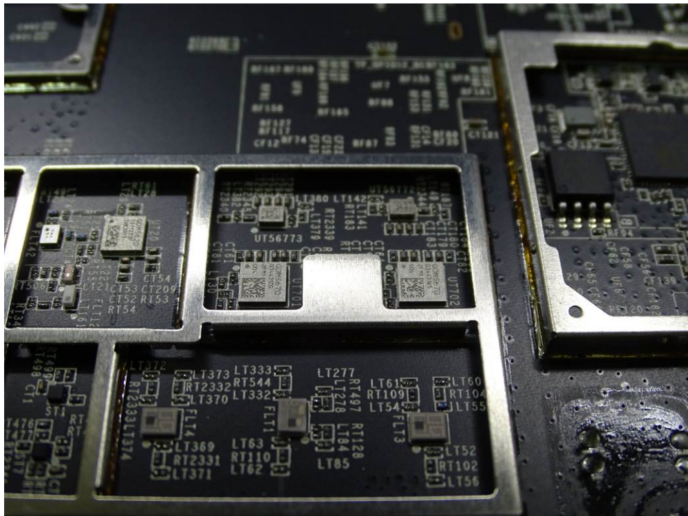
(86) EUT Photo
