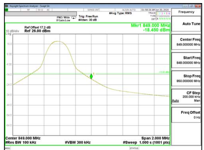
EDGE-ENDC_2A_n5-QPSK_10M(1,51)_CH168800_844
