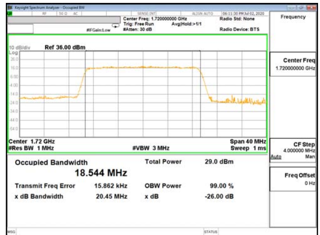
OCC-ENDC_66A_n5-QPSK_20M_CH132072_1720(100,0)
