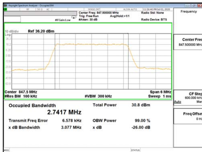
OCC-ENDC_5A_n2-QPSK_3M_CH20635_847.5(15,0)
